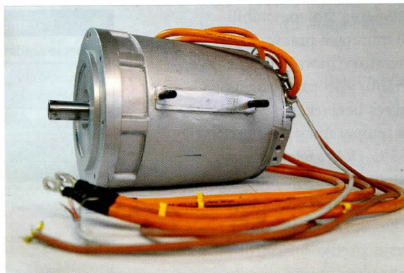
Rys. 2. Silnik synchroniczny z magnesami trwałymi SMKwsg132L-6C
