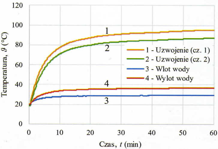
Rys. 4. Temperatury uzwojenia silnika podczas próby nagrzewania dla P_m = 60 kW, n = 4200 obr./min
