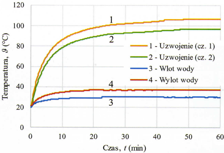
Rys. 3. Temperatury uzwojenia silnika podczas próby nagrzewania dla P_m = 60 kW, n = 3500 obr./min
