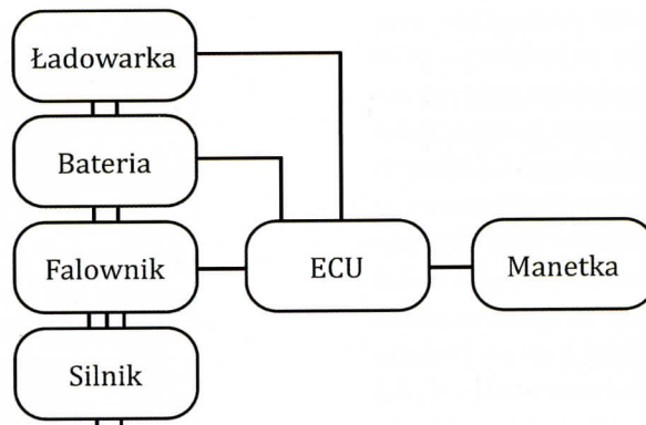
Rys. 1. Schemat blokowy układu napędowego
