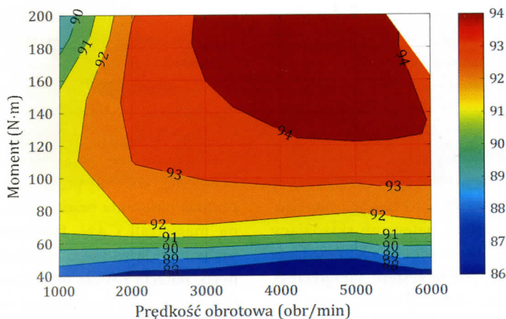
Rys. 5. Mapa sprawności silnika
