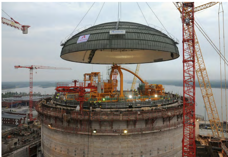
Rys. 5. Kopuła płaszcz metalowego obudowy reaktora EPR w elektrowni jądrowej Olkiluoto 3. Zdjęcie: Areva/TVO [11]
